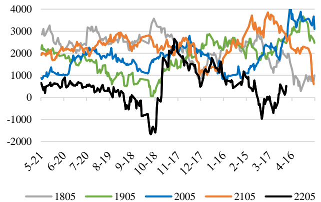
图表 38: 江苏醋酸利润率
