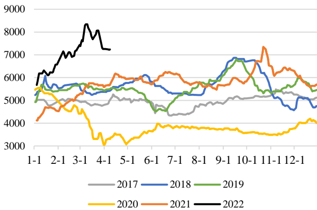
图表 52: MTBE 山东市场价
