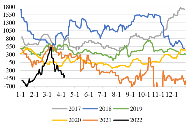
图表 27：陕西样本煤制企业现金流
