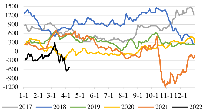
图表 29: 山东样本煤制企业现金流
