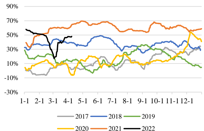
图表 40: 河南二甲醚利润率
