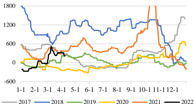
图表 30: 西南样本天然气制企业现金流
