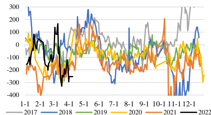
图表 34: 非伊甲醇进口利润
