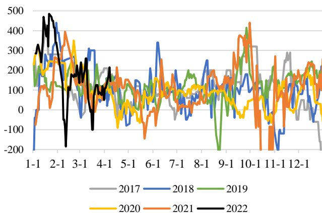
图表 56: 甲醇鲁北-关中价差
