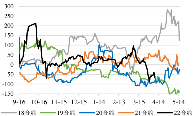
图表 44: 甲醇 05-09 价差
