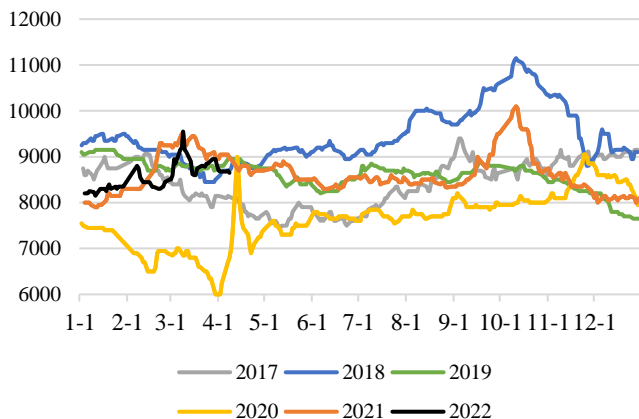
图表 50: 乙二醇华东市场价
