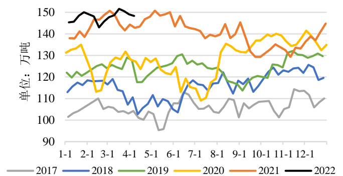
图表 3：甲醇周度产量
